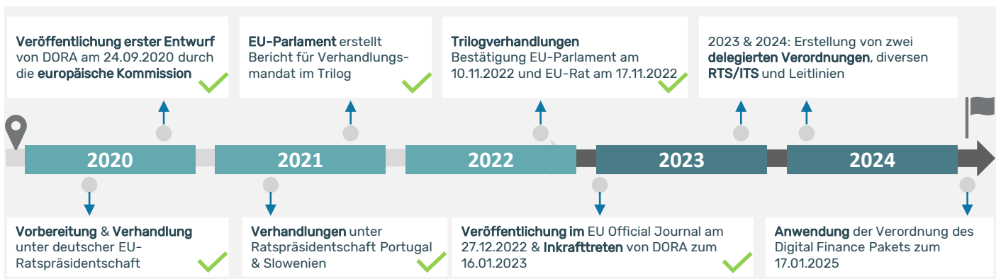
Abb. 1: Die DORA-Zeitschiene
